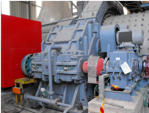
درایو کامل آسیاب غلطکی شامل کوپلینگ، موتور و گیربکس کمکی
