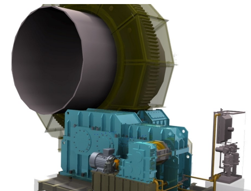
مدل سه بعدی از درایو کامل مربوط به کوره دوار (پروژه جایگزینی)
